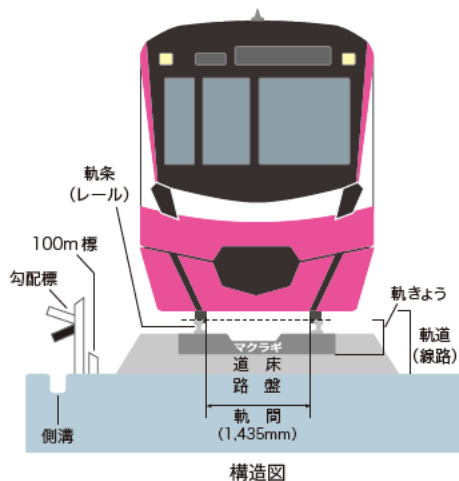
構造図
