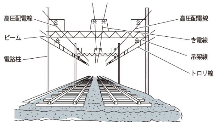
電路設備図
